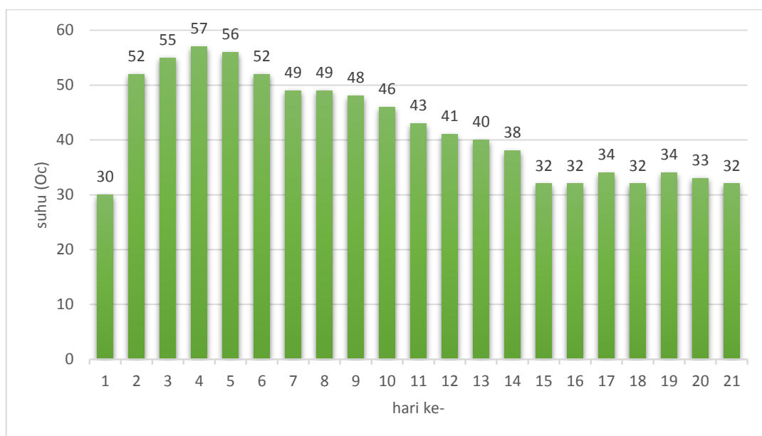
Gambar 4. Diagram Batang Suhu Tumpukan Kompos (°C) Selama Penelitian
