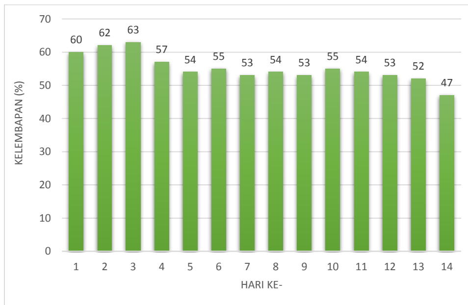
Gambar 5. Diagram Batang Kelembapan Tumpukan Kompos Eceng Gondok
