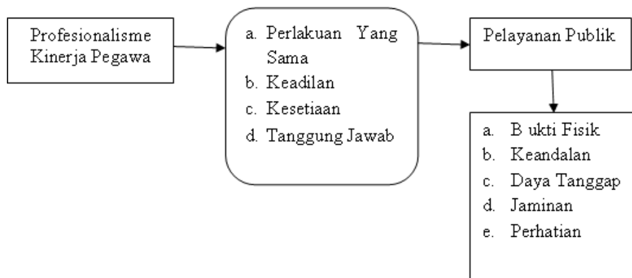
Gambar 1 Kerangka Konseptual
