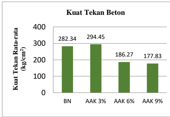
Gambar 4.1 Grafik Perbandingan Nilai Kuat Tekan Beton
