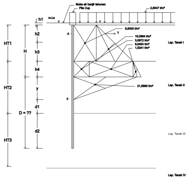
Gambar 4.2 Diagram Tekanan Tanah Aktif
