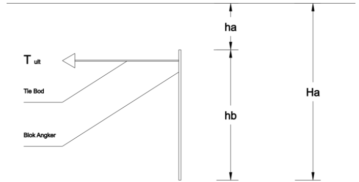
Gambar 4.8 Blok Angker
