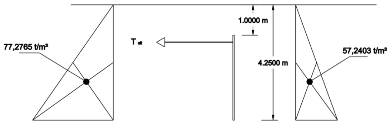
Gambar 4.9 Tekanan Tanah Aktif dan Pasif Pada Blok Angker
