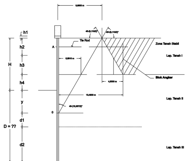
Gambar 4.7 Jarak Blok Angker Pada Metode Ujung Bebas
