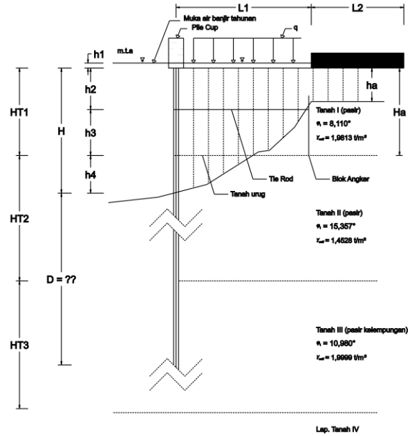
Gambar 4.1 Desain Konstruksi Sheet Pile
