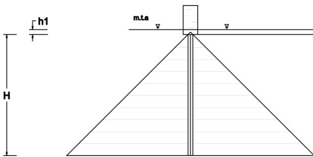
Gambar 4.3 Tekanan hidrostatik saling meniadakan
