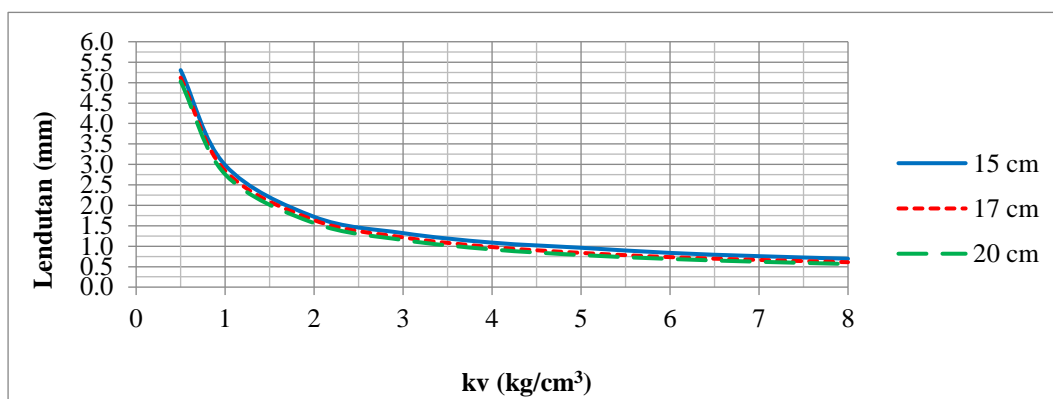
Gambar 8 Perhitungan lendutan Sistem Pelat Terpaku dengan koperan untuk beban 112,5 kN
