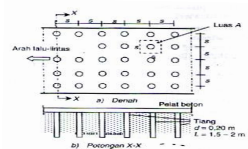
Gambar 2 Sistem Pelat Terpaku
